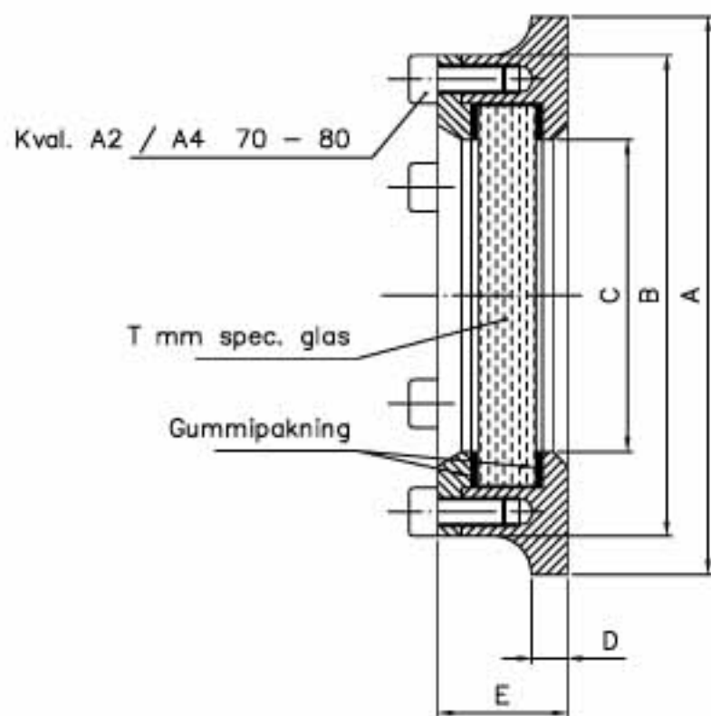
DIMENSION / DATATABEL FOR SKUEGLAS
